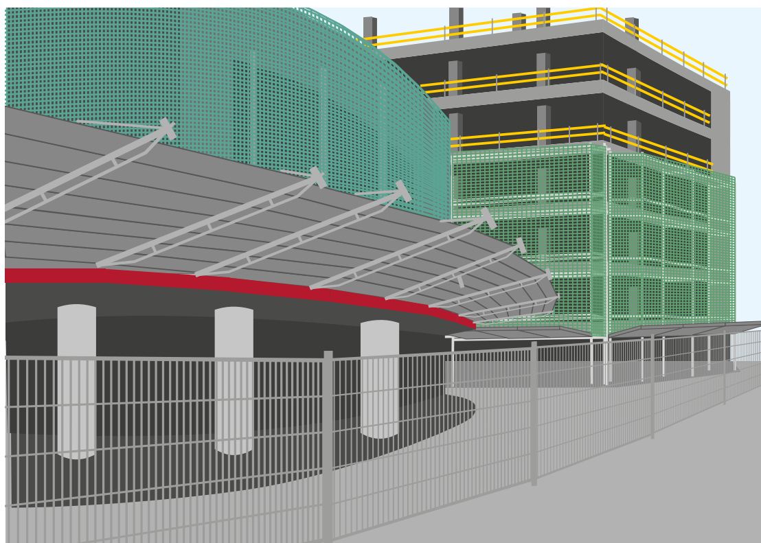
Rys. 4. Daszki ochronne
